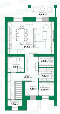
Планировочное решение №2 Первый этаж
